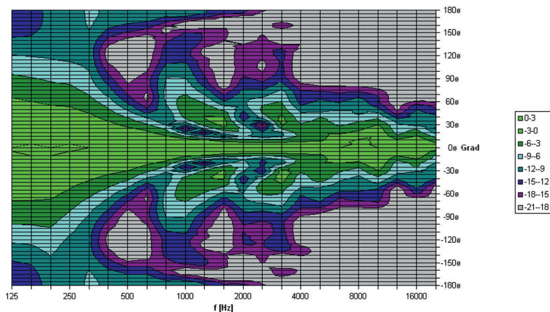
RL 204 SN vert. Direktivity Plot
