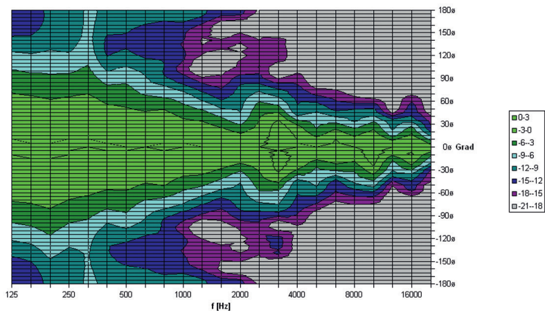
RL 204 SN hor. Direktivity Plot
